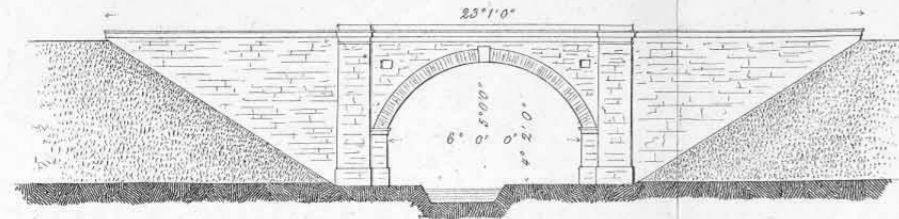
Ansicht der steinernen Brücke über den Hämrbach bei Mürzzuschlag.
