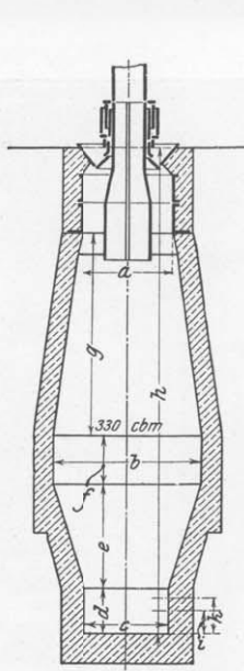
Fig. 56. Ofen Nr. 4.
