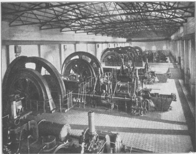
Kraftwerk A auf der Eisenhütte I.
