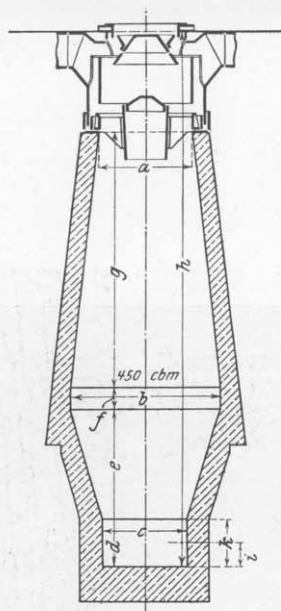
Fig. 53. Ofen Nr. 1.
