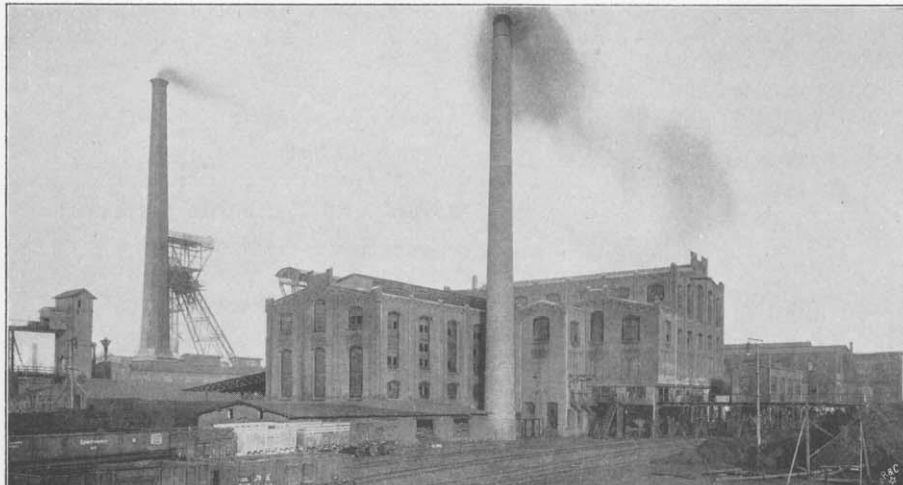
Figur 11, Zeche Oberhausen: Separation, Wäsche und Brikettfabrik.
