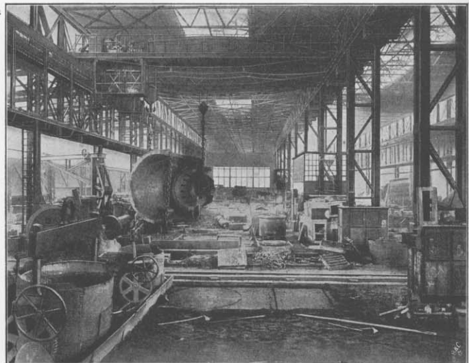
Figur 115. Gießerei: Innenansicht.
