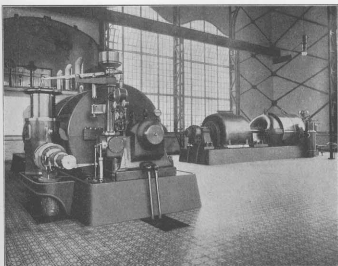
Zwei Hochdruck-Turbodynamos von je 2000 KW.
