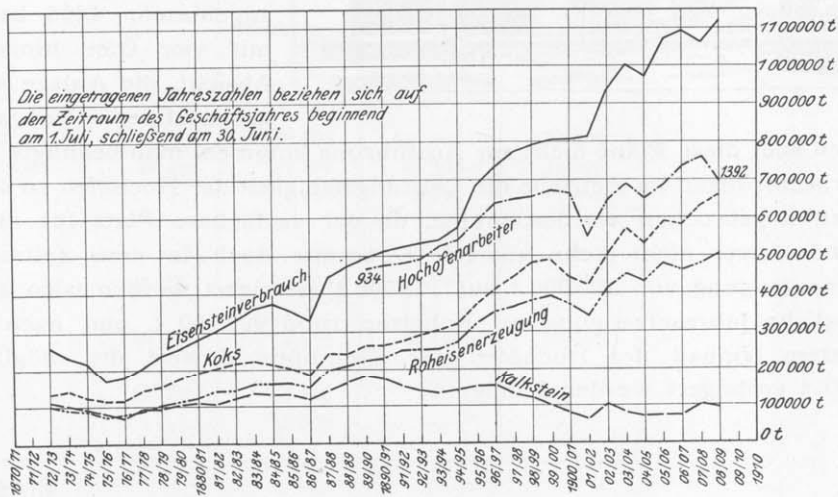
Figur 46. Anwachsen der Roheisenerzeugung.
