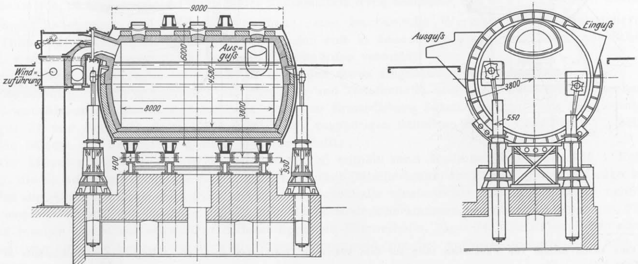
Figur 79 und 80. Roheisenmischer für 900 t-Roheiseneinsatz.
