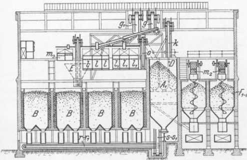
Figur 17: Schnitt J—K (Wäsche)
