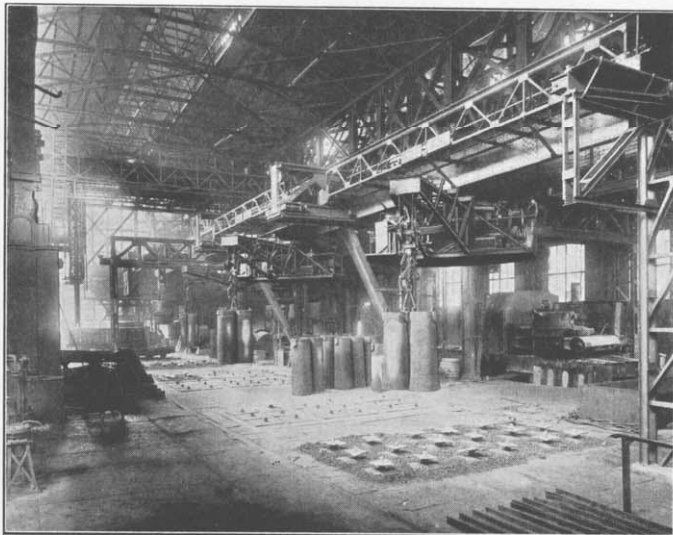
Tiefofenhalle mit Zangen-Laufdrehkranen.
