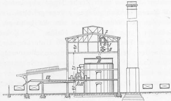
Figur 20: Schnitt P—Q (Brikettfabrik)
