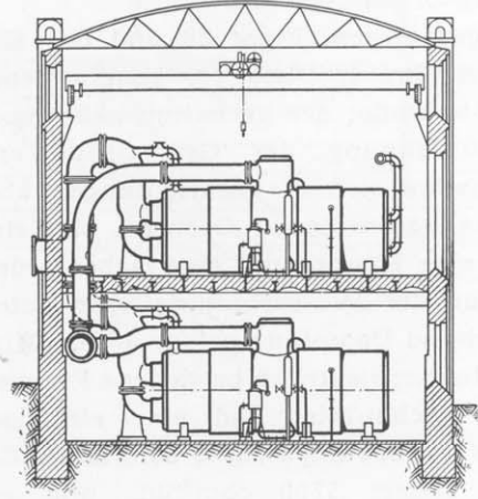
Figur 24, Schnitt a—b.
