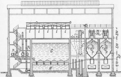
Figur 18: Schnitt L—M (Wäsche)
