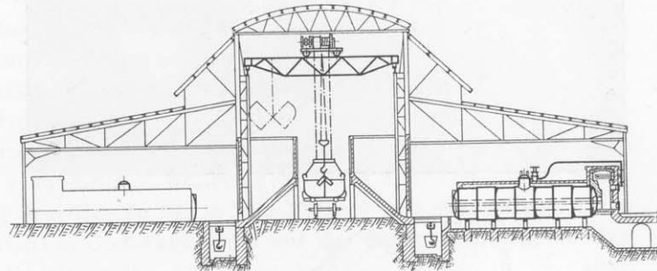
Figur 77. Schnitt g—h.
