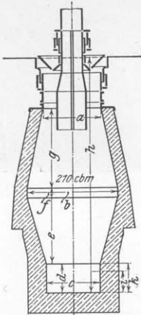
Fig. 60. Ofen Nr. 8.
