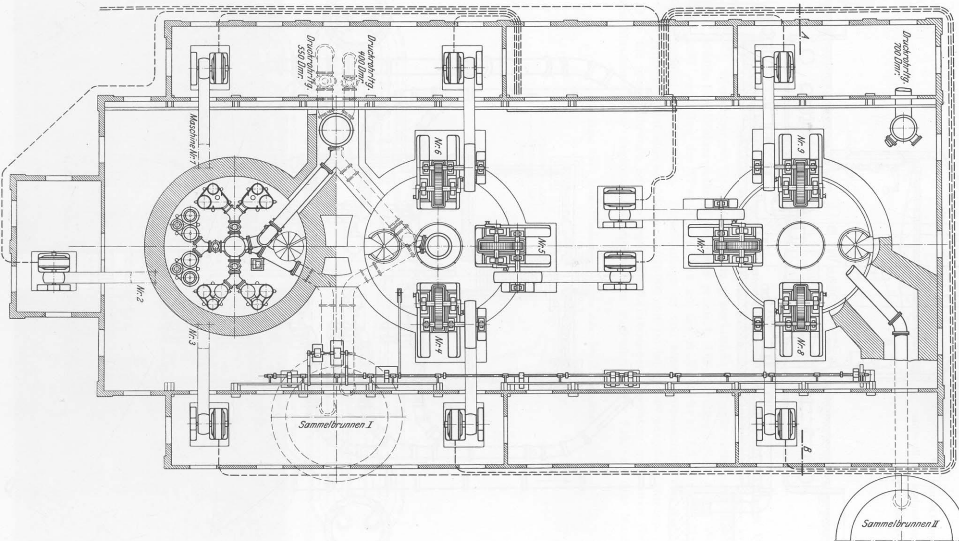
Figur 133. Pumpmaschinenanlage des Ruhr-Wasserverkes: Grundriß.
