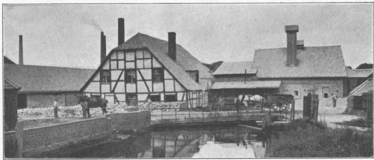
Figur 138. Steinfabrik Hammer Neu-Essen: Turbinen- und Kollerganghaus.
