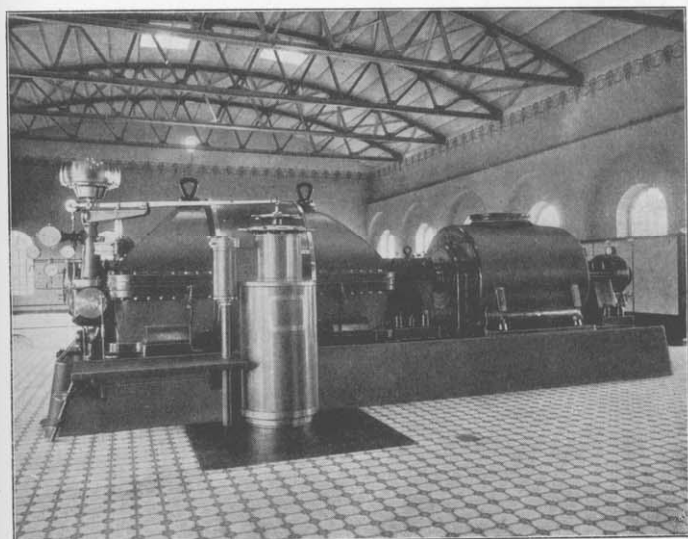
Abdampf-Turbodynamo von 1600 KW.
