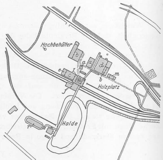
Figur 28, Zeche Hugo: Lageplan der Tagesanlagen.
