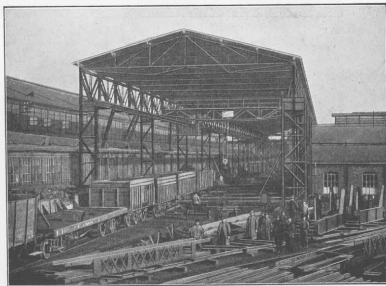
Figur 128. Brückenbauabteilung: überdeckte Kranbahn.
