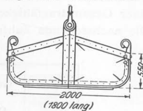
Figur 149. Erzkübel.
