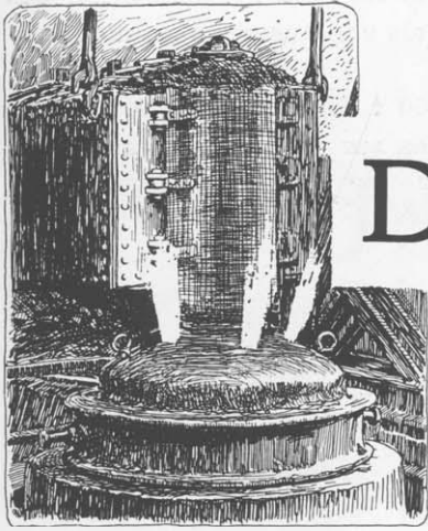
Figur 116. Stahlformgießerei: Innenansicht.
