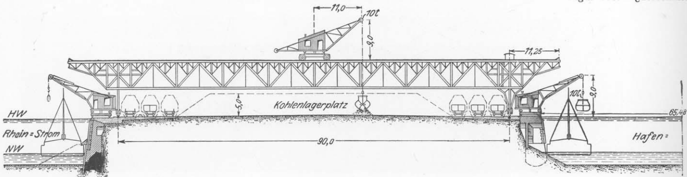
Figur 155. Querschnitt
