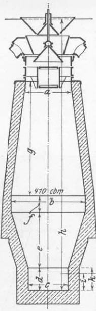
Fig. 54. Ofen Nr. 2.
