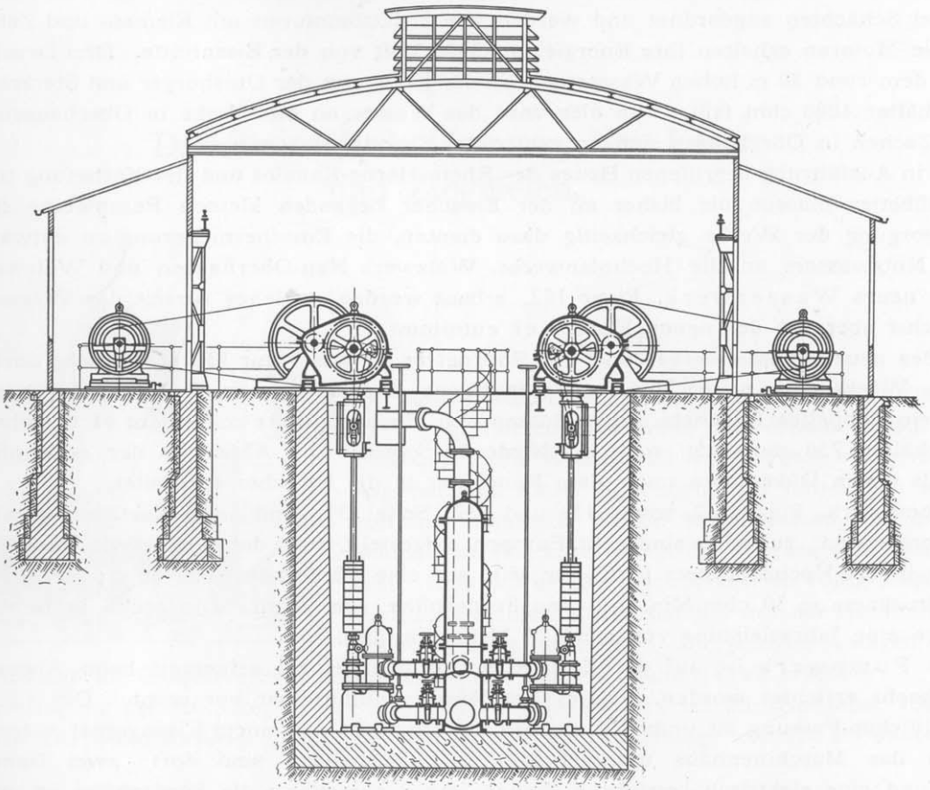
Figur 134. Pumpmaschinenanlage des Ruhr-Wasserwerkes: Aufriß.
