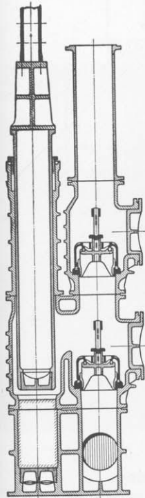
Figur 108. Maßstab 1:100.
