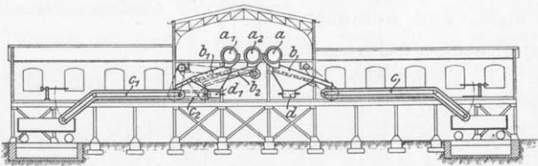
Figur 13: Schnitt A—B (Aufbereitung)
