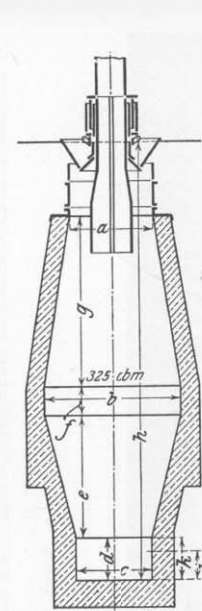
Fig. 58. Ofen Nr. 6.
