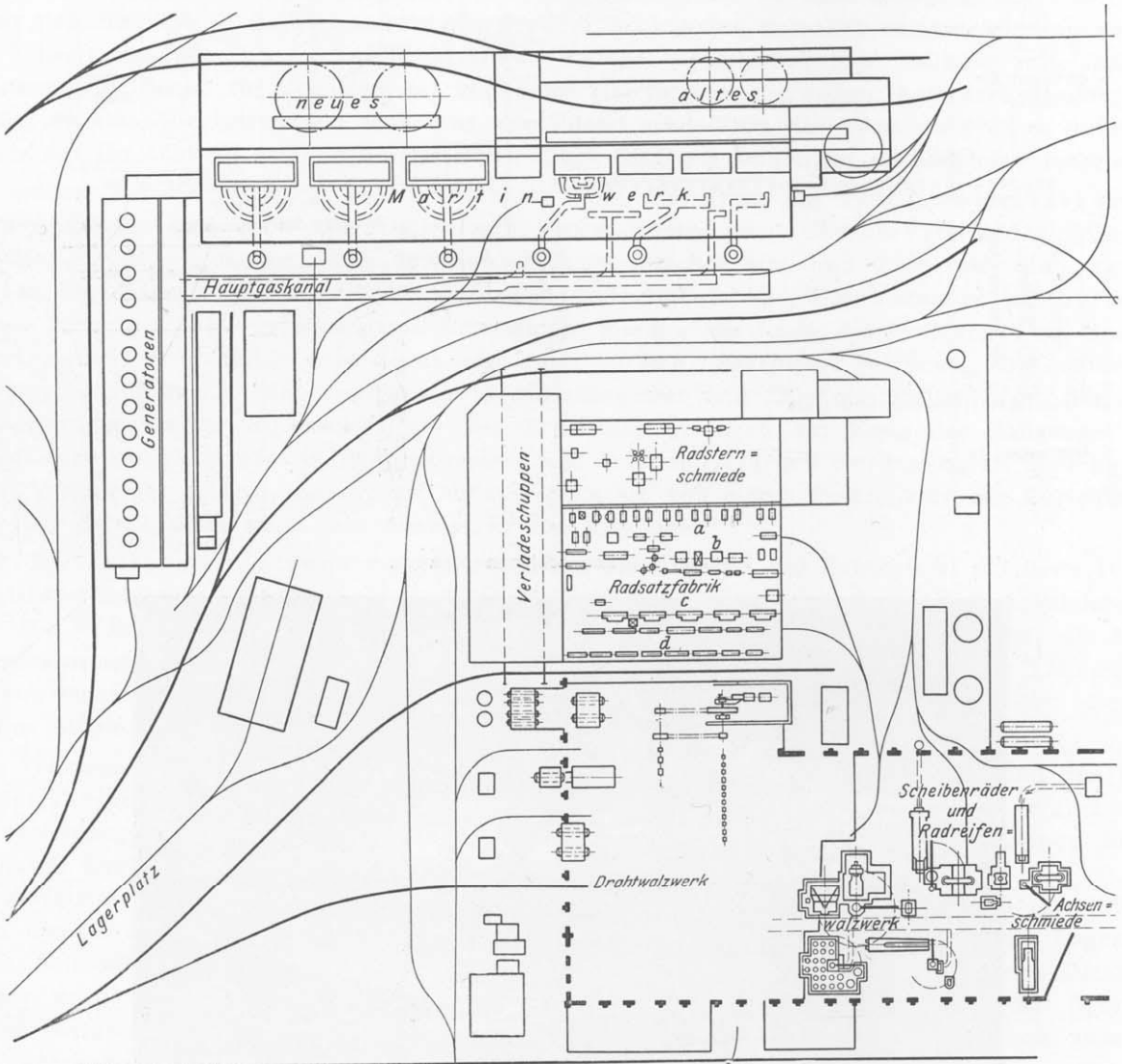
Figur 90. Neues Martinwerk.
