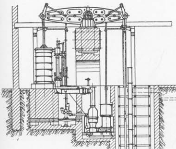
Figur 107. Maßstab 1:500.
