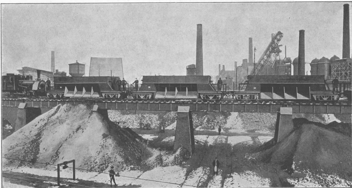
Fig. 146. Entladen der Talbot-Erwagen von der Hochbahn auf die Erzhalde.
