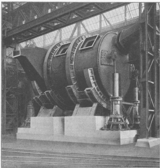
Figur 81. Roheisenmischer.
