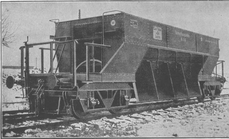
Figur 145. 50 t-Talbotscher Selbstentladewagen für Erz.
