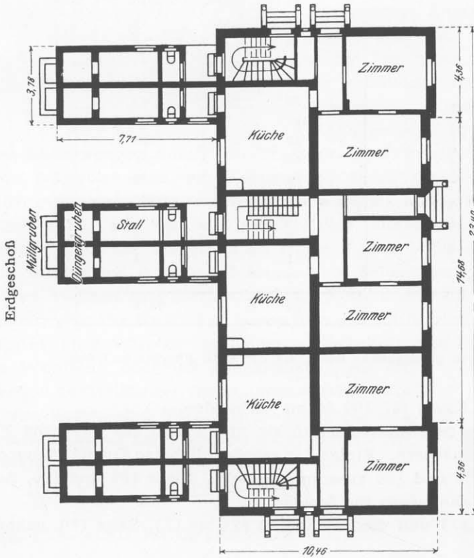
Figur 159 und 160. Sechsfamilien-Arbeiterwohnhaus, ausgeführt in den Kolonien der Zeche Ludwig, Gerschermannshof und Hiesfeld.
