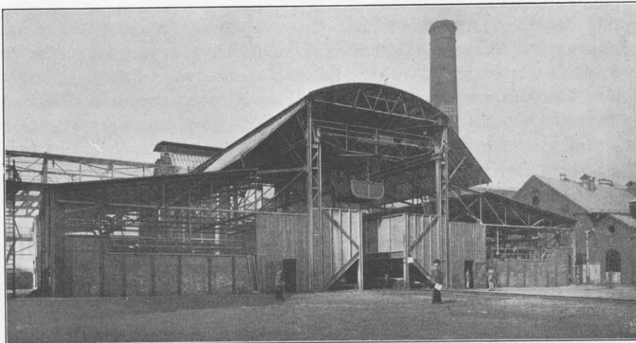
Figur 92. Kesselanlage mit Kohlebunkern.
