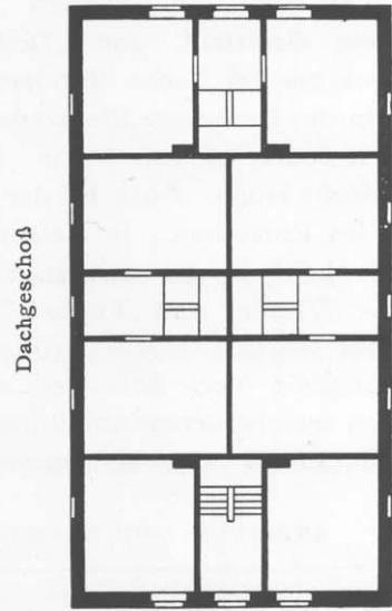
Figur 161 und 162. Vierfamilien-Arbeiterwohnhaus, ausgeführt in den Kolonien Stemmersberg, Eisenheim und Dunkelschlag.
