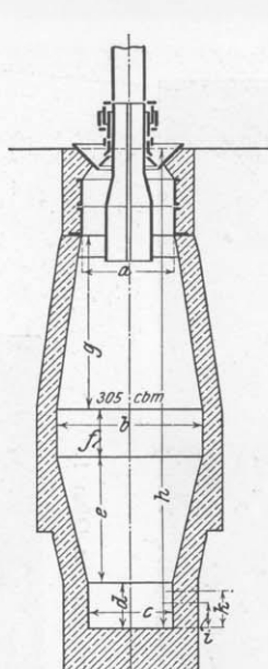
Fig. 55. Ofen Nr. 3.
