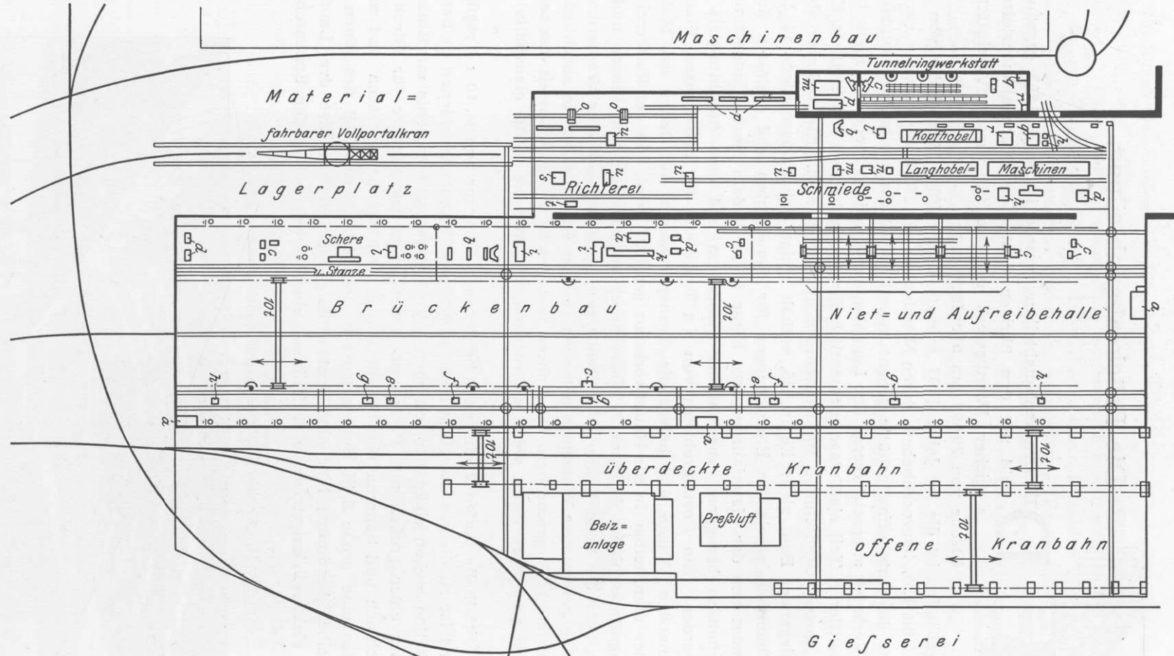
Figur 125 und 126 Haupthalle der Brücken- baubereitung.
