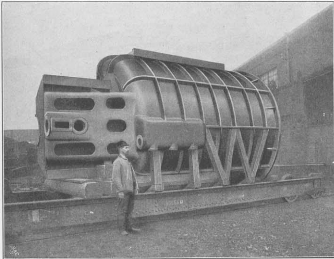
Hinteres Unterteil eines Schiffsturbinengehäuses.
