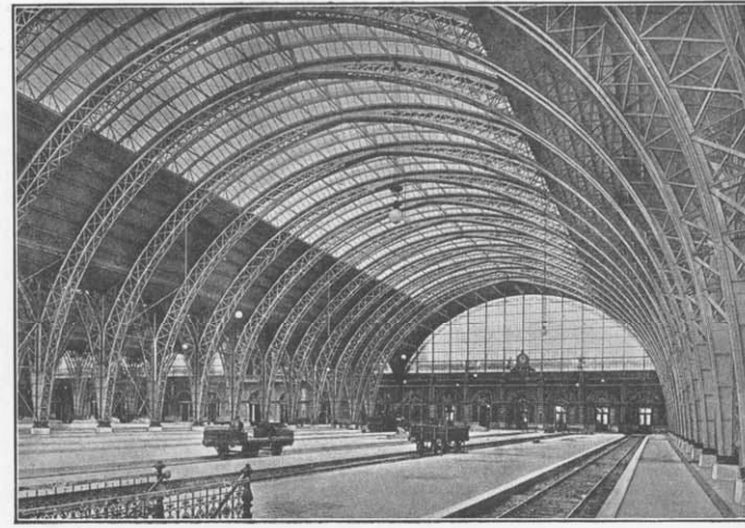
Halle des Hauptbahnhofes zu Frankfur a. M.
