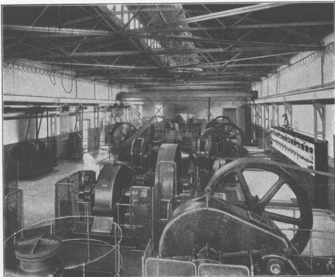
Figur 131. Ruhr-Wasserwerk an der Ackerfähr.
