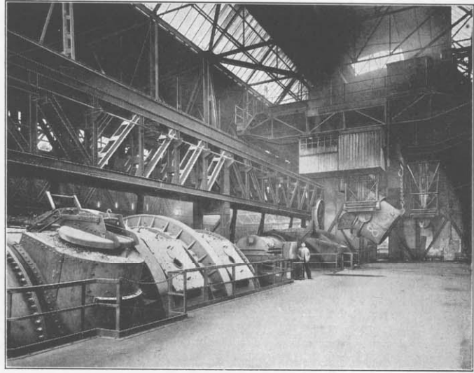
Entleeren der Roheisenpfannen in den Mischer.
