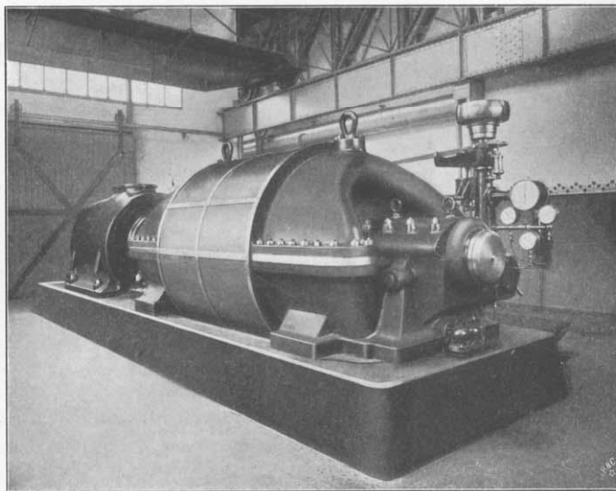
Kraftwerk F auf Walzwerk Neu-Oberhausen.
