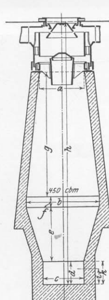
Fig. 57. Ofen Nr. 5.
