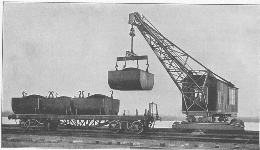
Figur 150. Kokskübelwagen.
