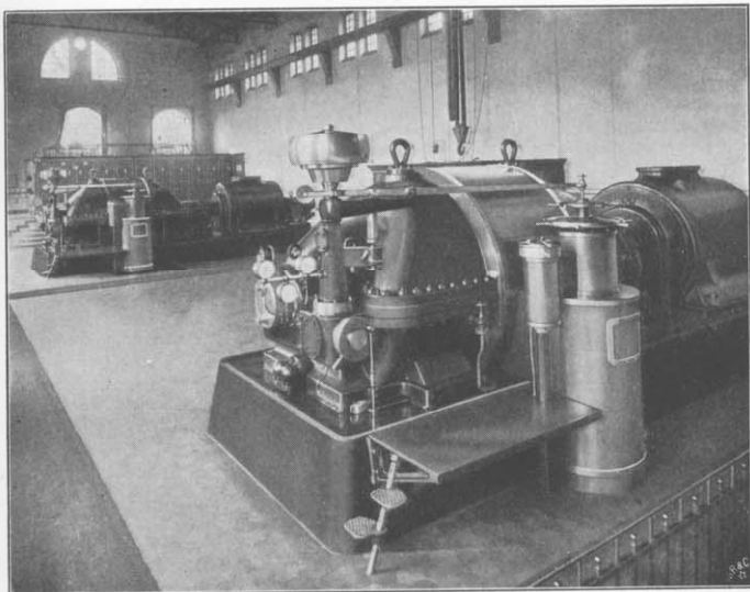
Kraftwerk C auf Zeche Osterfeld.
