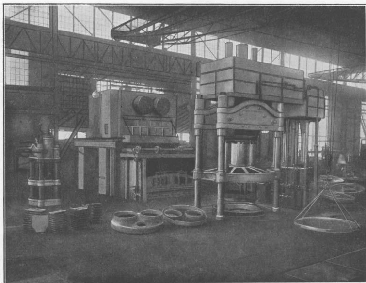
Figur 100. Kumpelpresse.
