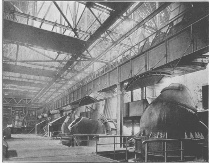
Birnenhalle.
