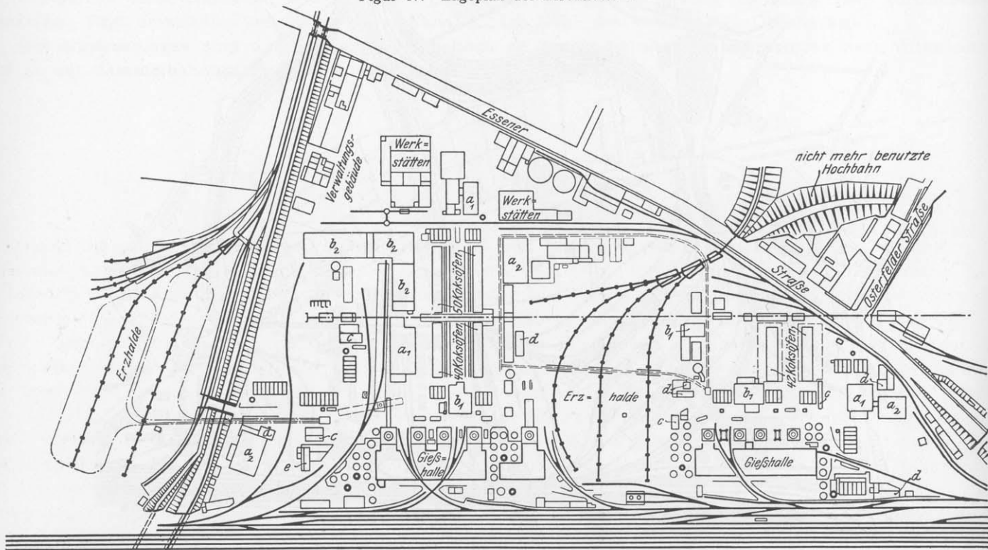
Figur 47. Lageplan der Eisenhütte I.
