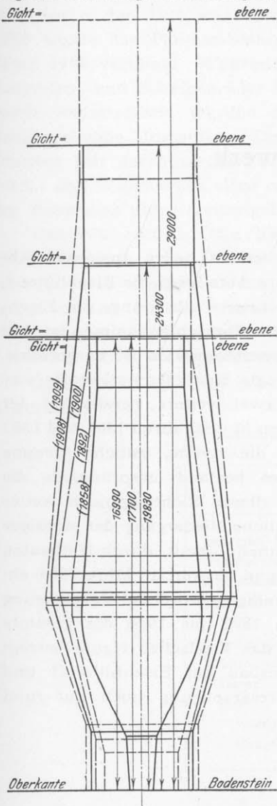
Fig. 45. Entwicklung der Hochofenprofile.
