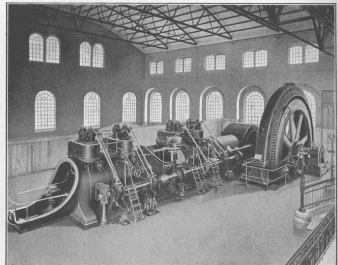
Doppeltwirkende Viertakt-Gasmaschine für Dynamoantrieb.
