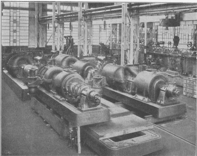
Turbo-Dynamos im Zusammenbau.
