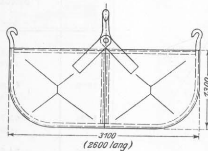
Figur 149. Erzkübel.
