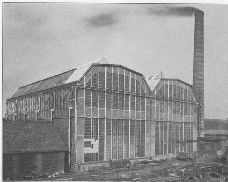
Figur 123. Turbinenfabrik: Außenansicht.
