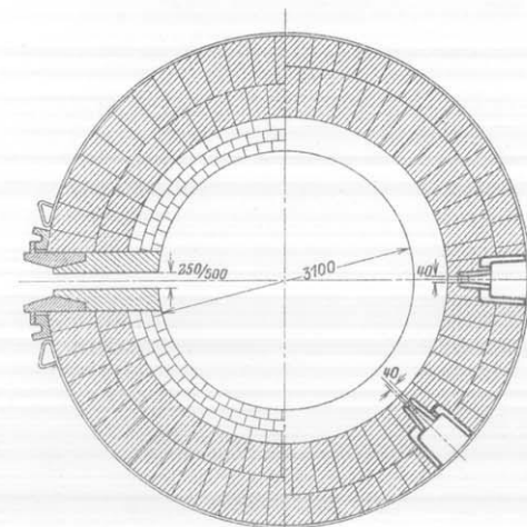
Schnitt durch Eisenabstich Schlackenformen
