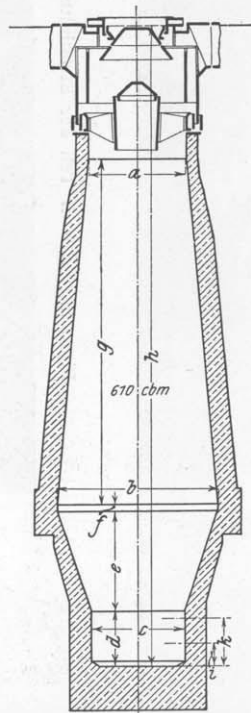
Fig. 62. Ofen Nr. 10 u. 11.
