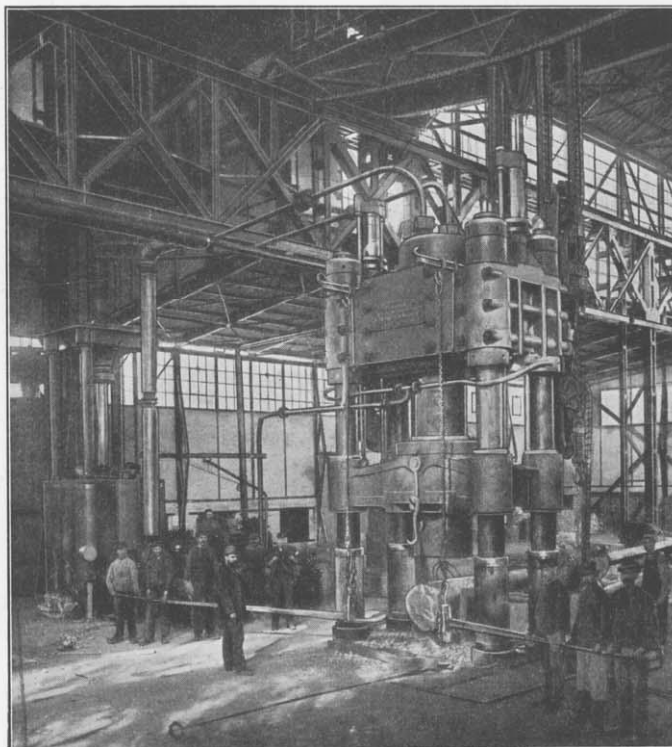
Figur 121. Preßwerk: 2500 t-Pressen.
