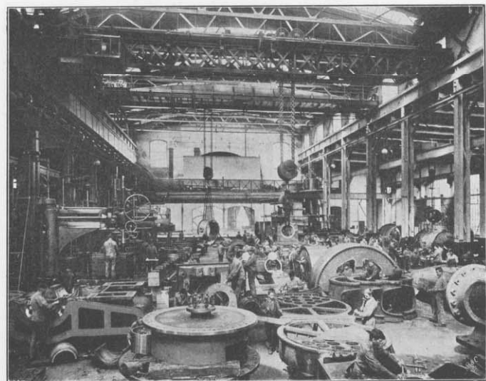
Montagewerkstatt.
