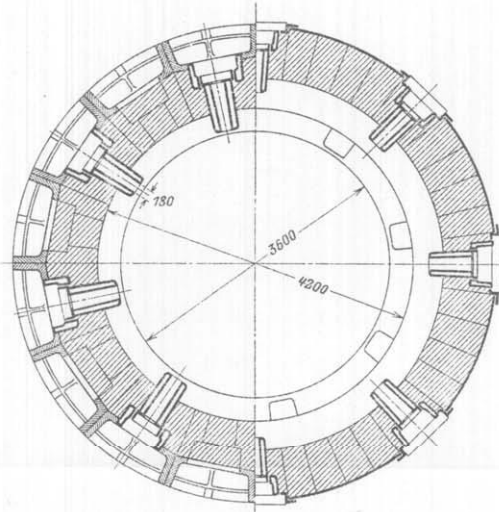
Schnitt durch Windformen Notwindformen
