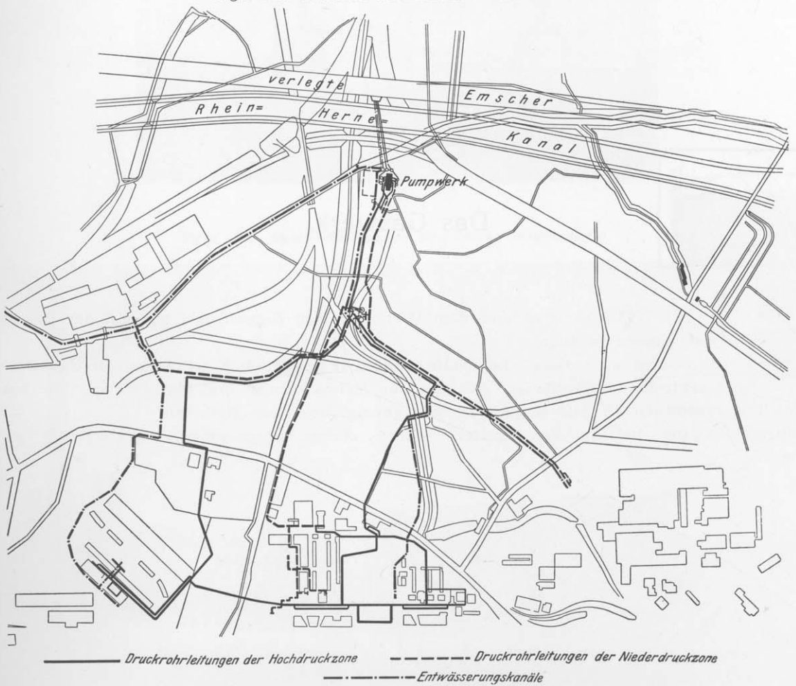
Figur 135. Rohrnetz des Emscher-Wasserwerkes.
