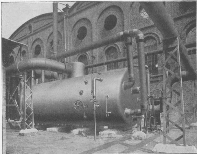
Wärmespeicher-Anlage.
