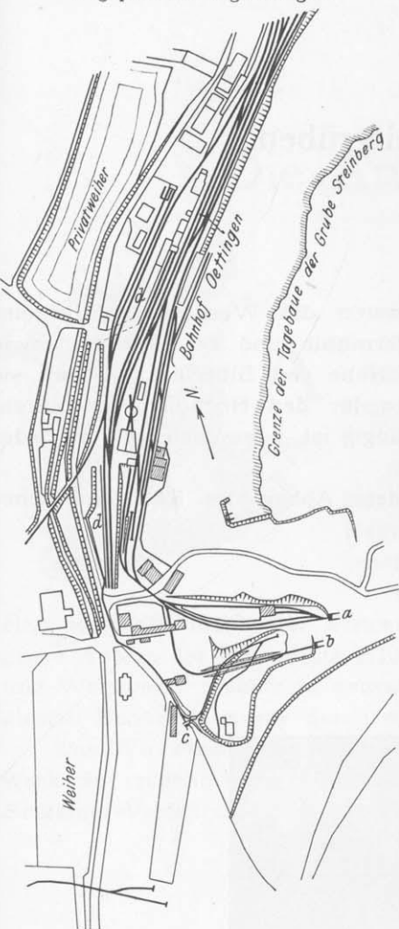
Figur 40. Eisensteingruben Steinberg, Sterkrade-Anschluß und Sterkrade-Anschluß II: Lageplan der Tagesanlagen.
