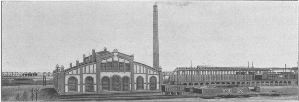
Zeche Vondern (Kokerei und Gasmaschinen-Kraftwerk).
