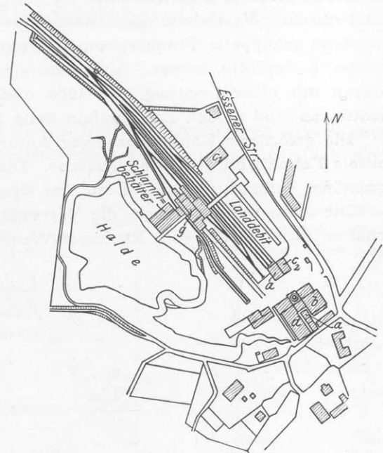
Figur 31, Zeche Ludwig: Lageplan der Tagesanlagen.
