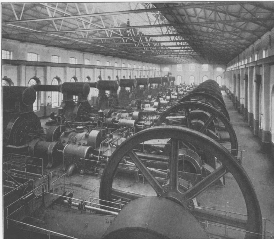
Figur 69. Gichtgas-Gebläsemaschinenhaus.
