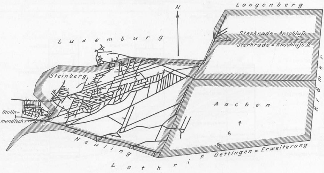
Figur 39. Eisensteingruben Steinberg, Sterkrade-Anschluß und Sterkrade-Anschluß II: Abbau auf dem grauen Lager.
