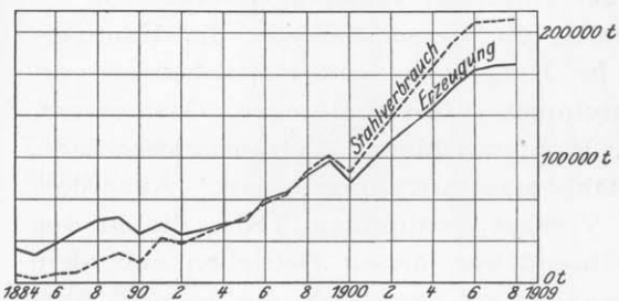
Figur 105. Stahlverbrauch und Gesamterzeugung des Walzwerkes Oberhausen.
