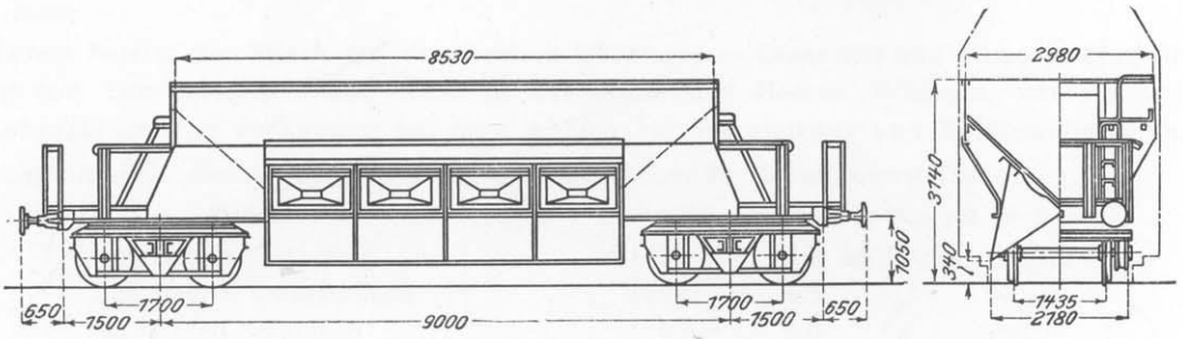
Figur 143 und 144. 50 t-Talbotscher Selbstentladewagen für Erz.
