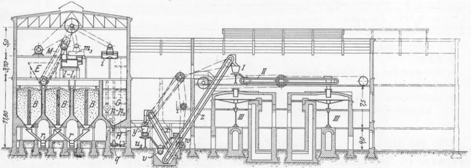
Figur 16: Schnitt G—H (Wäsche und Brikettfabrik)
