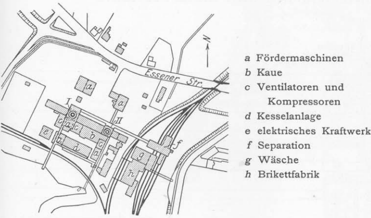
Figur 9, Zeche Oberhausen : Lageplan der Tagesanlagen.
