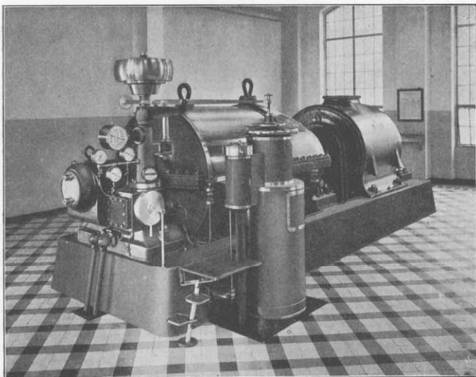
Abdampf-Turbodynamo von 900 KW.
