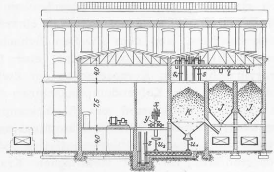
Figur 19: Schnitt N—O (Wäsche)
