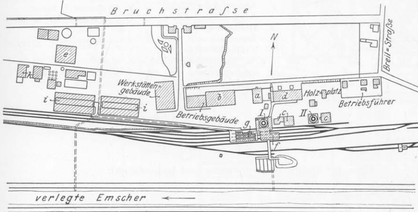
Figur 21, Zeche Vondern: Lageplan der Tagesanlagen.
