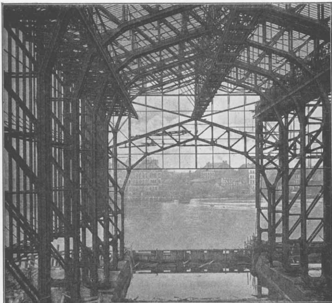
Überdachte Helling der Germaniawerft in Kiel.
