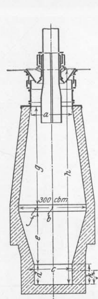
Fig. 59. Ofen Nr. 7.
