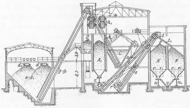
Figur 15: Schnitt E—F (Wäsche)
