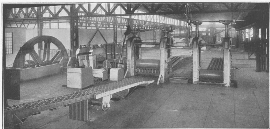
Figur 99. Grobblechwalzwerk: Lauthsches Triogerüst.
