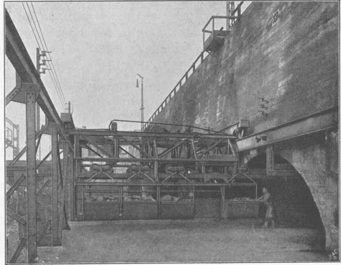
Erzschiebebühne.
