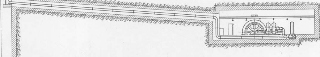
Figur 109. Maßstab 1:500.
