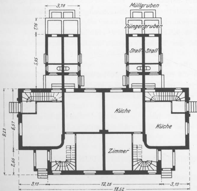
Figur 167 und 168. Vierfamilien-Arbeiterwohnhaus, ausgeführt in den Kolonien Vonderbruch und Hiesfeld.
