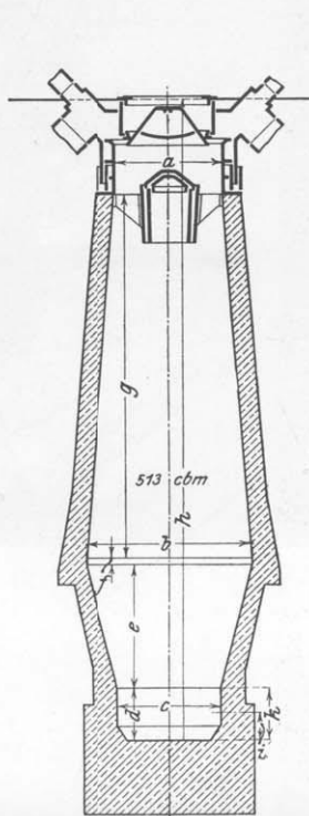
Fig. 61. Ofen Nr. 9.
